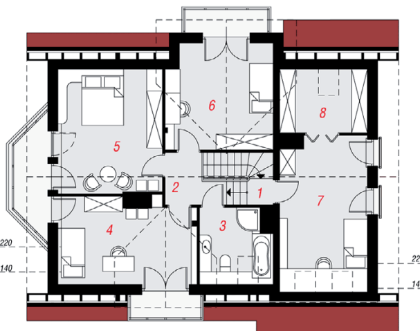
PODDASZE
