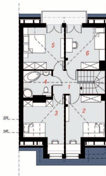
PODDASZE
