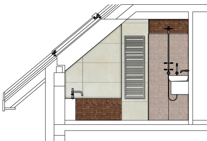
widok D/1:50
