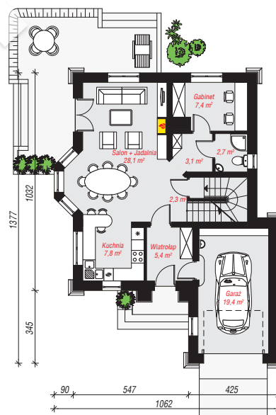
PARTER: 76,20 (0,00) m 2
