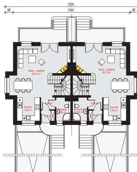
PARTER: 93,40 (0,00) m 2
