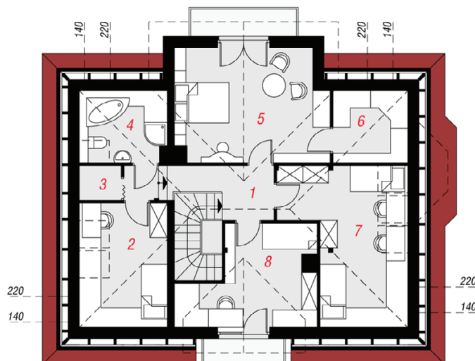
PODDASZE
